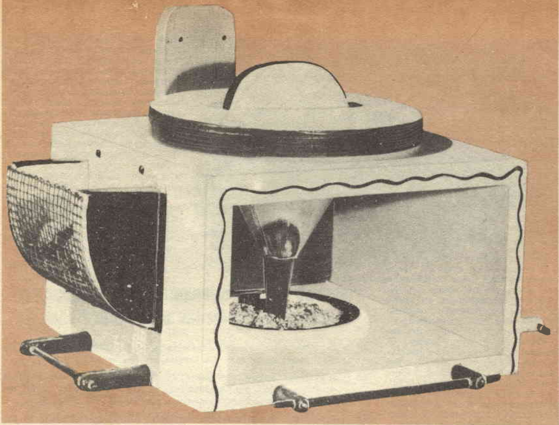
Una semplicissima versione di distributore; il serbatoio del beccime è rappresentato da un imbuto, il cui collo, serve da tramoggia, per la discesa dei semi, alla superficie della quale gli uccelli possono attingerli
