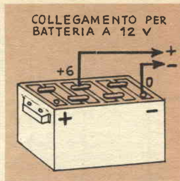
Circuito per il prelievamento della tensione di 6 volt da una batteria a 12, per l'alimentazione del ricevitore
