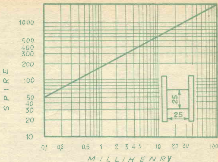
Filo da usare, mm, 0,8 od 1. La scala della colonna verticale si riferisce al numero delle spire da avvolgere sul supporto di mm. 25 di diametro, per ottenere un dato valore di induttanza in millihenries. Ad esempio, per ottenere una induttanza di 2 millihenries occorrono 270 spire circa. Le caratteristiche del supporto sono quelle illustrate nell'insero. L'anima cilindrica è di legno o cartone bachelizzato, di diametro 25 mm. larga pure 25 mm. Le fiancattine sono dischi di fibra o di cartone robusto. Evitare l'impiego di ferro e perfino di chiodi
