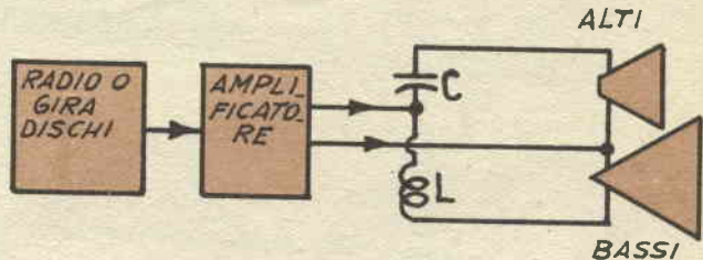
Schema per blocchi di un complesso caratteristico per bassa frequenza
