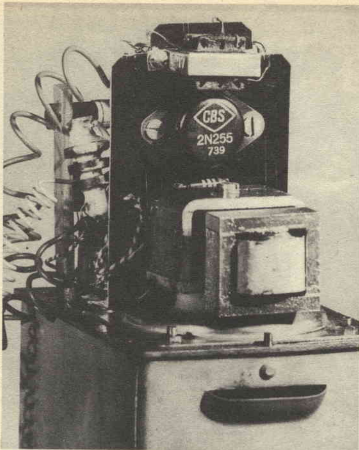
Veduta della parte superiore dello chassis dell'apparecchio: si nota, in basso, l'altoparlantino, con il trasformatore di uscita, al centro il transistor di potenza 2N255, ed in alto, il trasformatore di pilotaggio del transistor stesso, AR-96. L'apparecchio, in questa foto è realizzato nella versione professionale e tale può essere installato su di uno scooter o su di un'automobile
