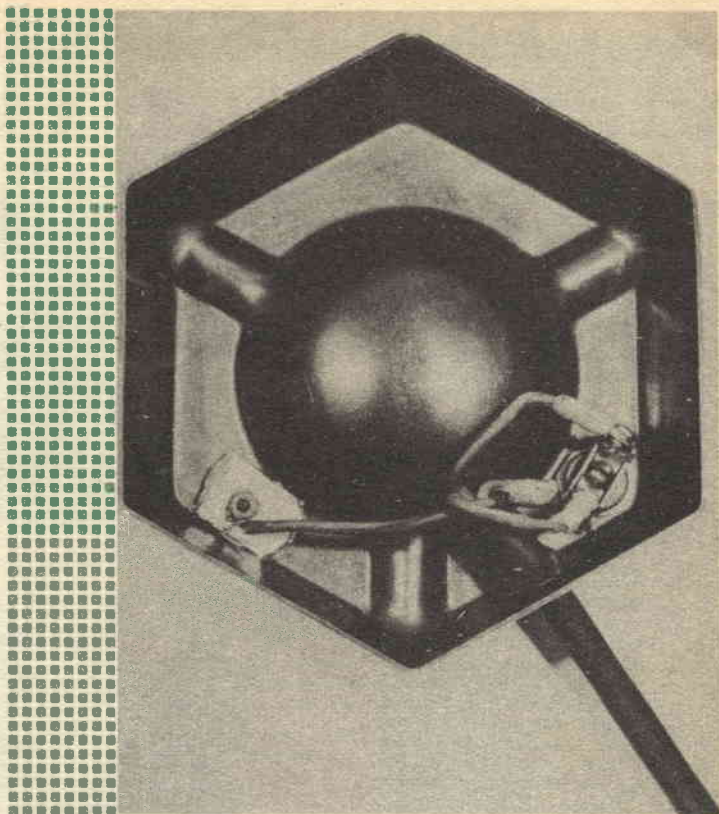
L'interno del portaceneri con i collegamenti al pulsante e quelli alla resistenza di accensione; a questa ultima giunge un solo filo perché l'altro è collegato alla massa del portaceneri, cosa possibilissima data la bassa tensione in giuoco. Notare la rondella di mica per il montaggio della resistenza per isolarne uno dei terminali
